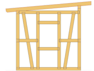
Fachwerk
